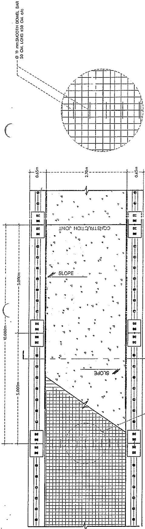
แบบขยาย B ขนาดจริง 1:50
