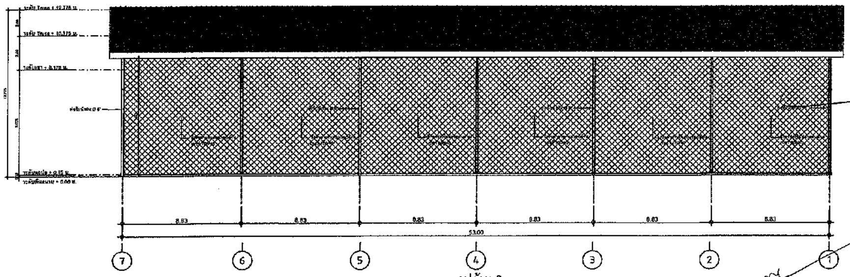
รูปตําน 3 มาตราส่วน 1:100
