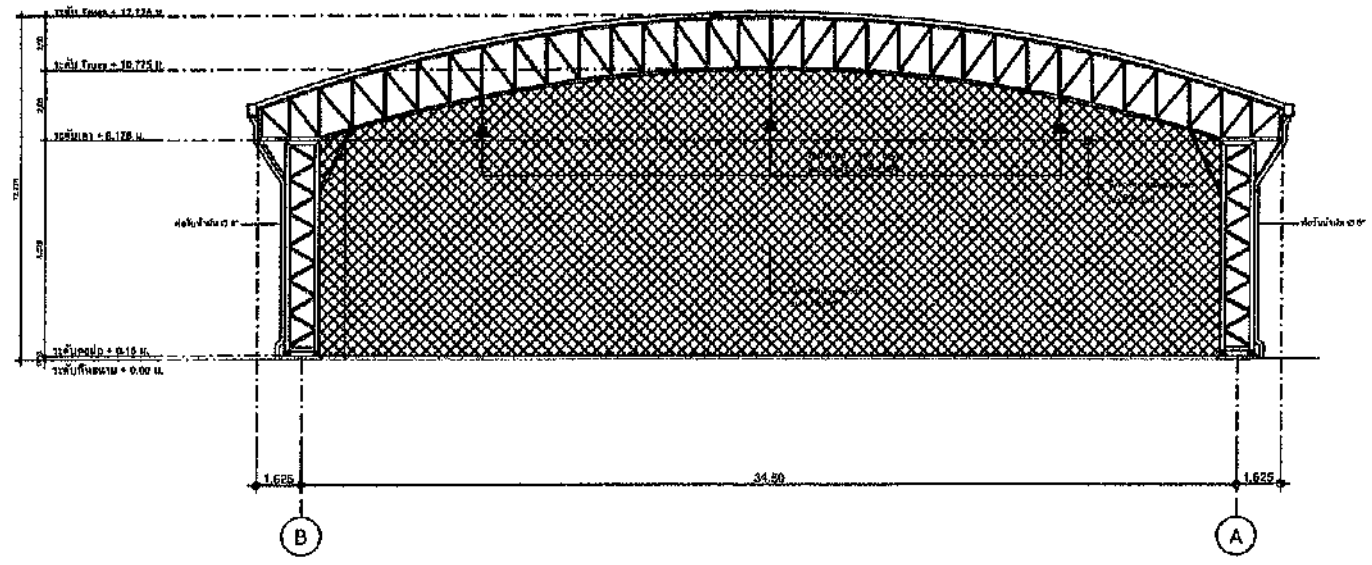
รูปด้าน 2 ขนาด 1:100
