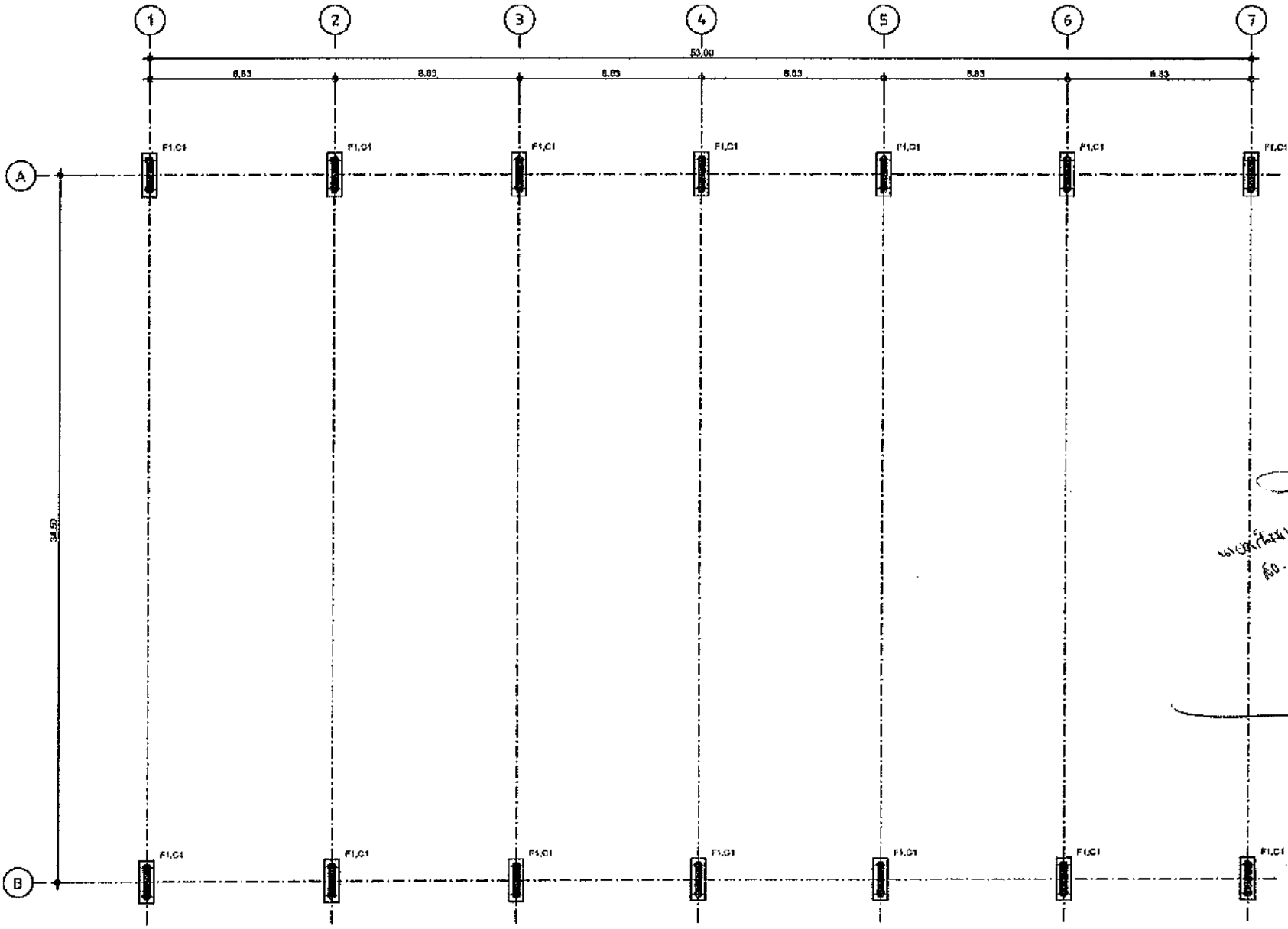
แปลนฐานราก เสาต่อมือ ขนาดจริง 1:100
