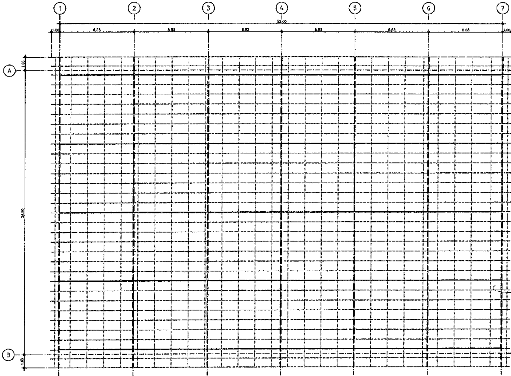
แปลนโครงสร้างรับหลังคา มาตราส่วน 1:100
