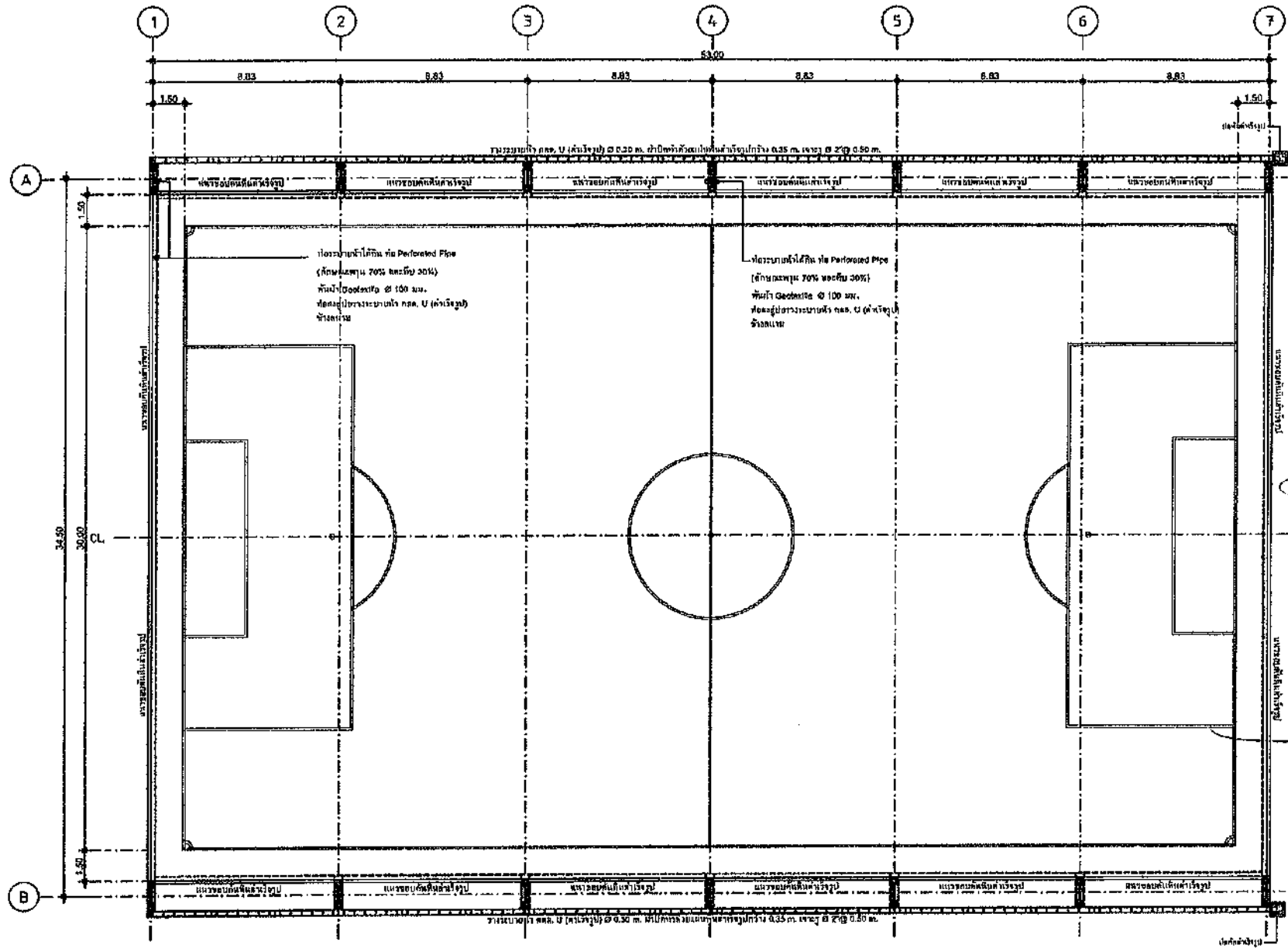
แบบแสดงแนวท่อระบายน้ำใต้ดินฟุตบอลหญ้าเทียม อาคารต่าง 1:100
