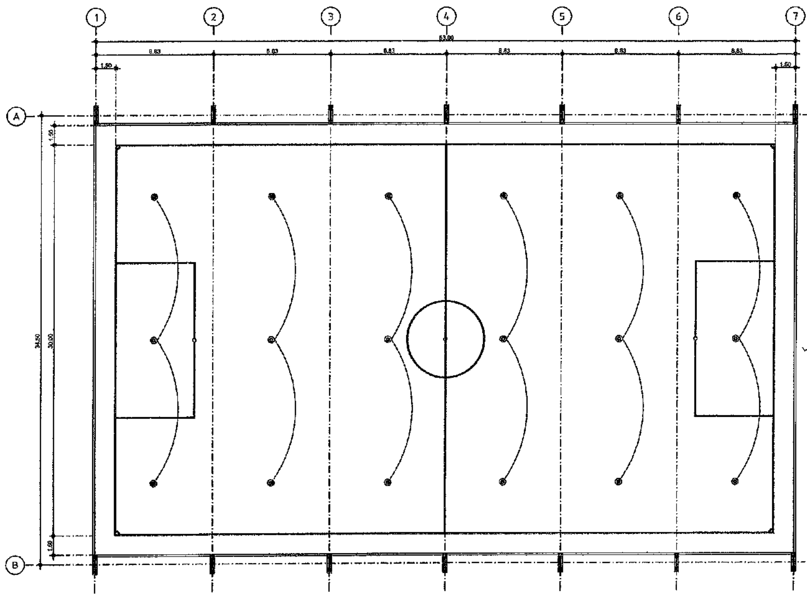
แบบแสดงตำแหน่งไฟฟ้าแสงสว่าง 1:100
