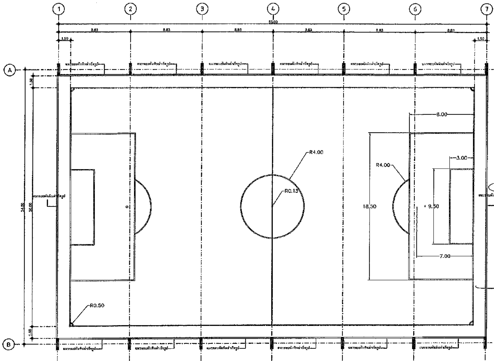
แบบแสดงสนามฟุตบอลหญ้าเทียม ขนาดกว้าง 33.00ม. ยาว 53.00 ม.
