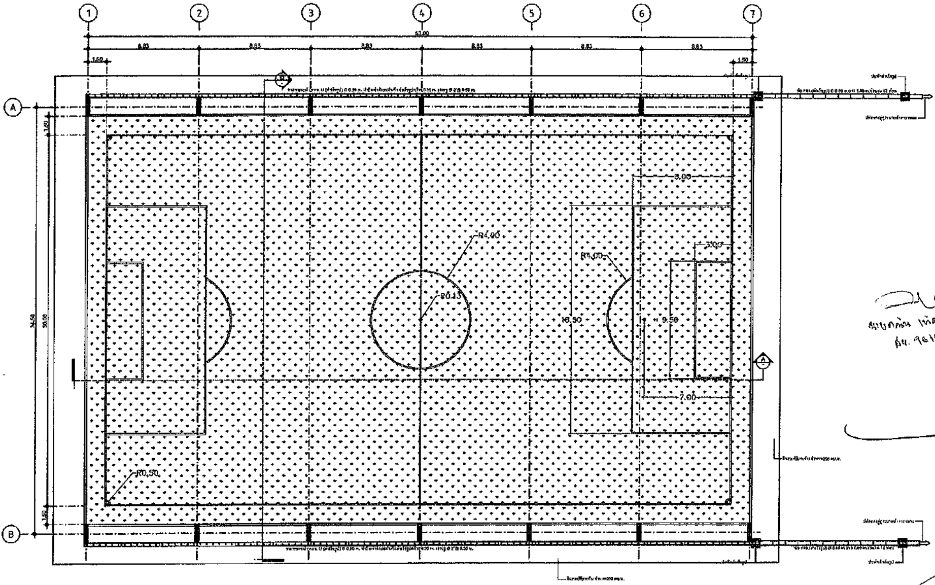
แปลนสนามฟุตบอลหญ้าเทียม ขนาดจริง 1:100
