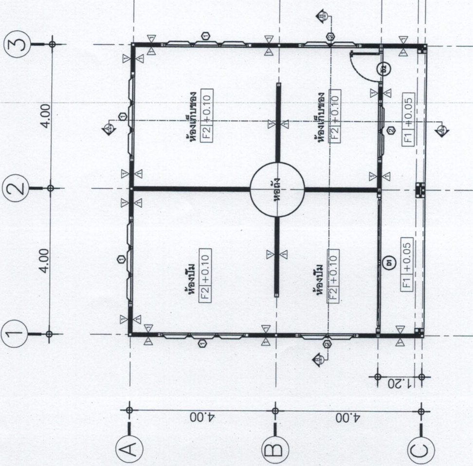
แปลนพื้นที่ห้อง 1:100
